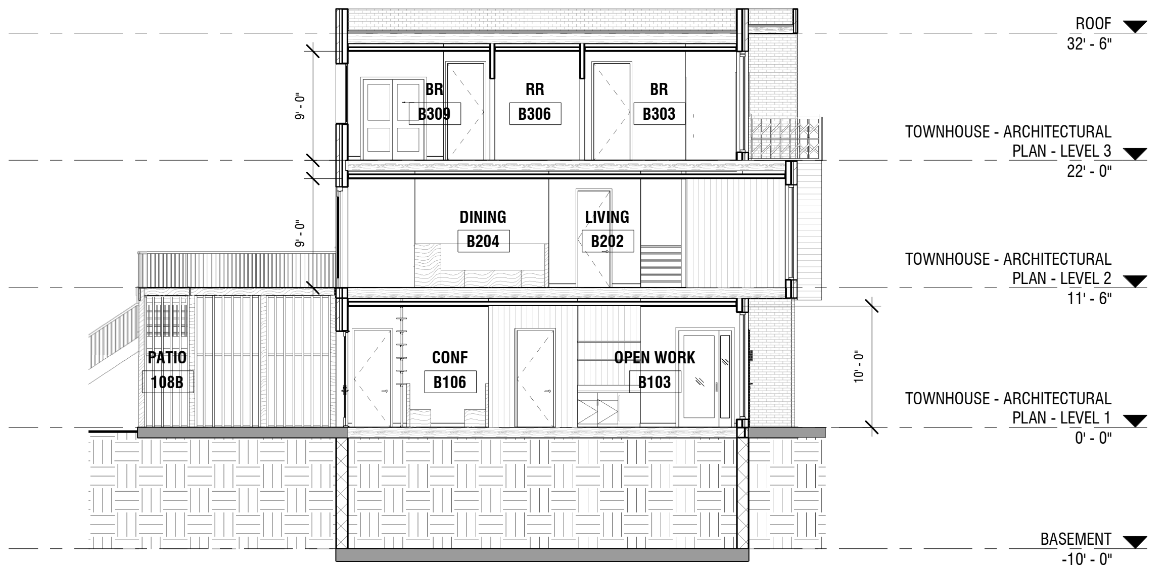
① TOWNHOUSE - LONGITUDINAL SECTION 1/8" = 1'-0"
